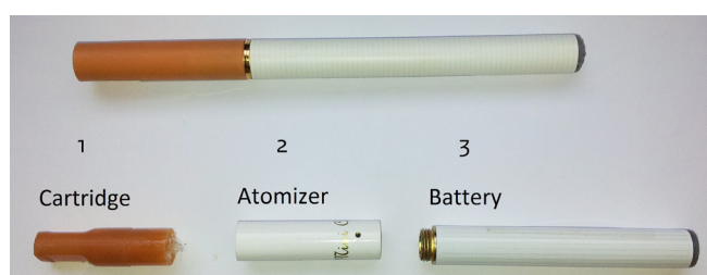
Figuur 1: componenten van een e-sigaret.
